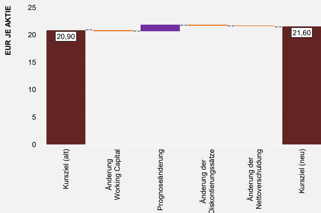
ABBILDUNG 1: WASSERFALLDIAGRAMM DER ANPASSUNGEN DES DCF-MODELLS
