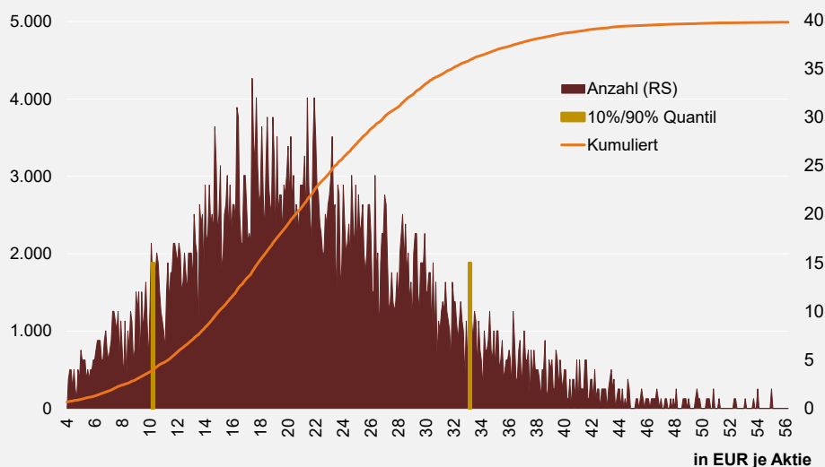
ABBILDUNG 2: HISTOGRAMM DER MONTE CARLO-SIMULATION
