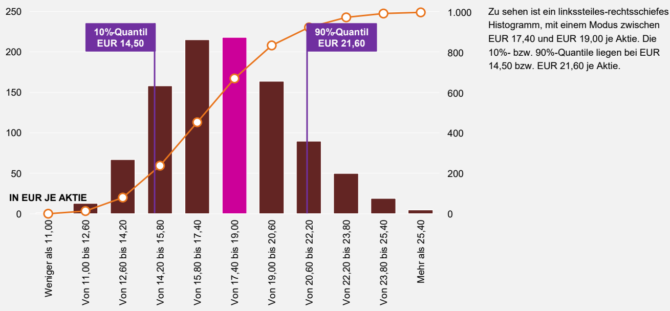
ABBILDUNG 1: MONTE CARLO-SIMULATION
