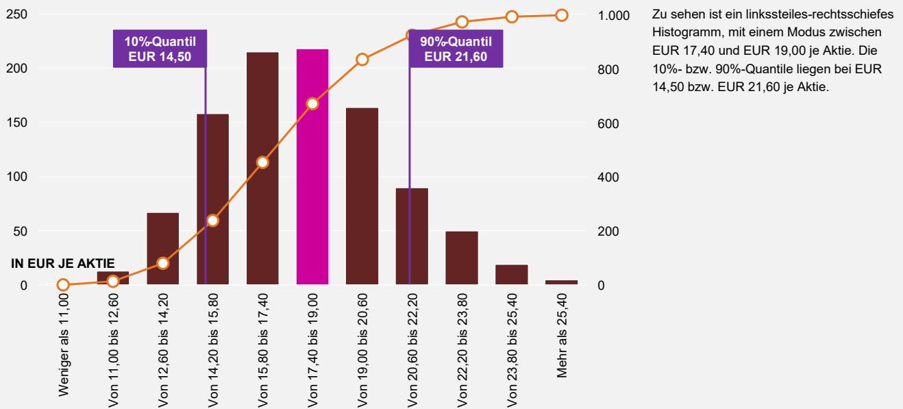
ABBILDUNG 1: MONTE CARLO-SIMULATION
