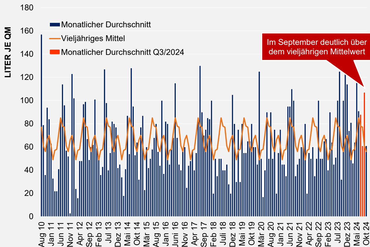
ABBILDUNG 1: NIEDERSCHLAGSMENGEN DEUTSCHLAND
