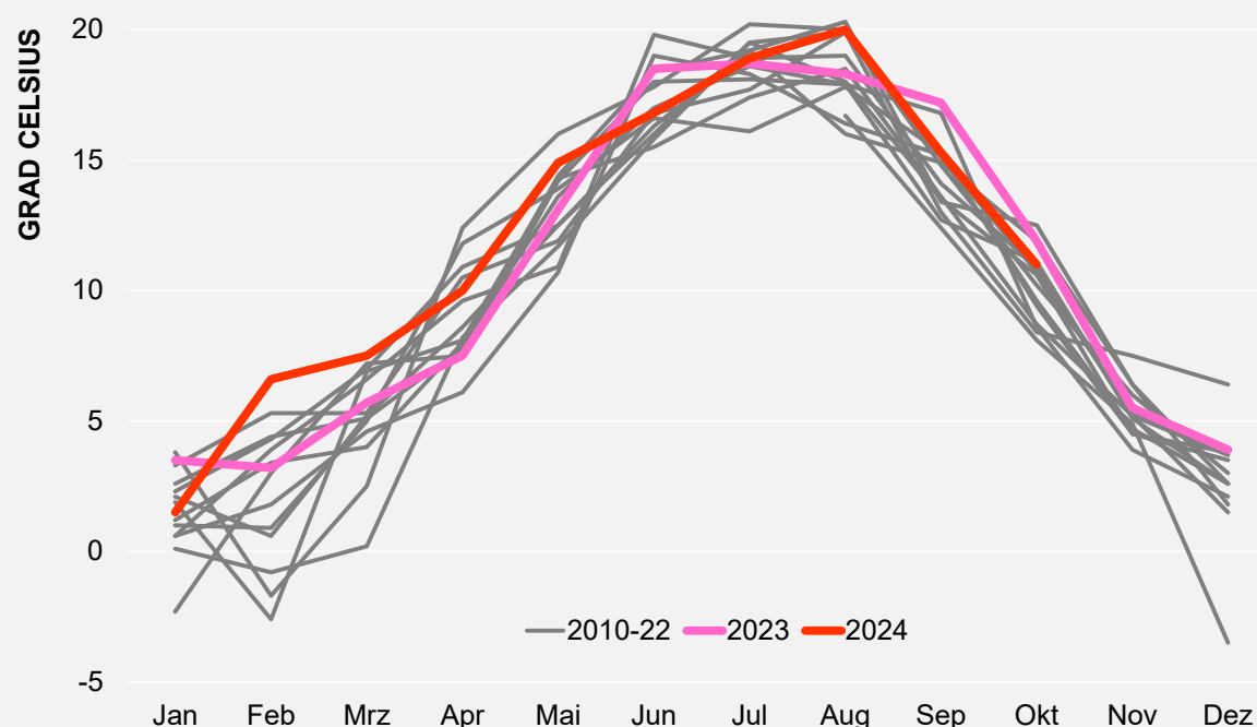
ABBILDUNG 2: DURCHSCHNITTSTEMPERATUREN DEUTSCHLAND
